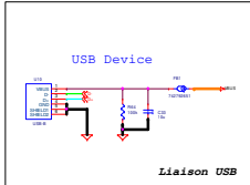
Liaison USB
