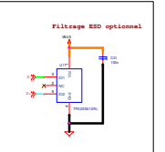
Liaison USB
